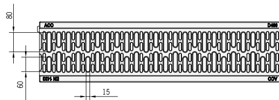
Wymiary kanału ACO Drain Monoblock PD 200V, 1,0 m
