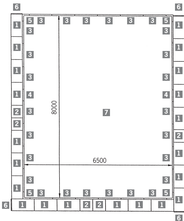
Plan ułożenia elementów łapacza piasku
