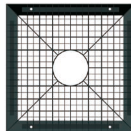
Boczna część z wyciętym otworem DN/OD 160
