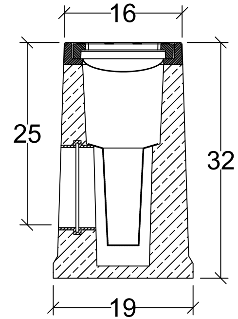
przekrój poprzeczny
