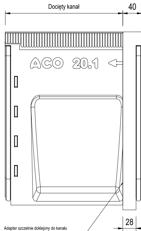
Przykład połączenia z docinanym kanałem
