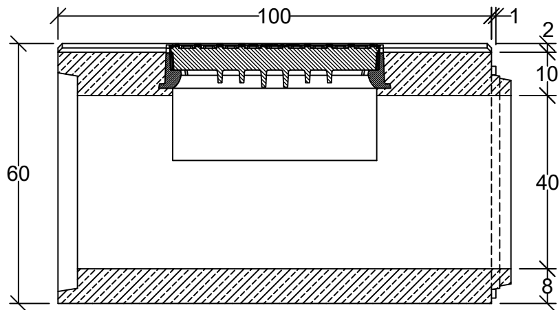
Pzekrój podłużny
