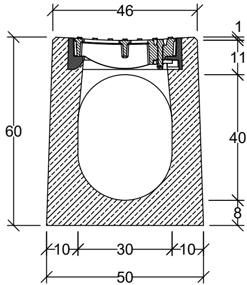
Przekrój poprzeczny
