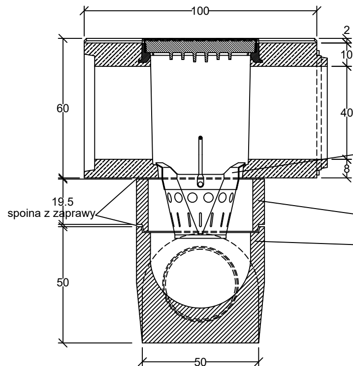
przekrój podłużny
