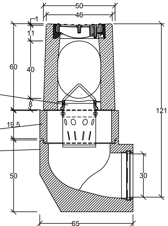
przekrój poprzeczny
