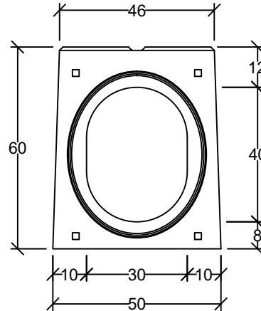
Widok króciec
