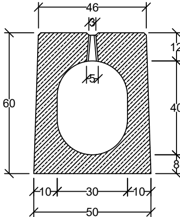
Przekrój
