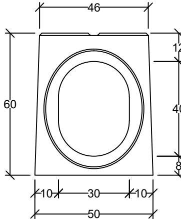
Widok gniazdo
