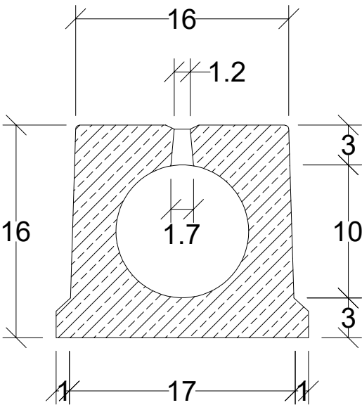
przekrój
