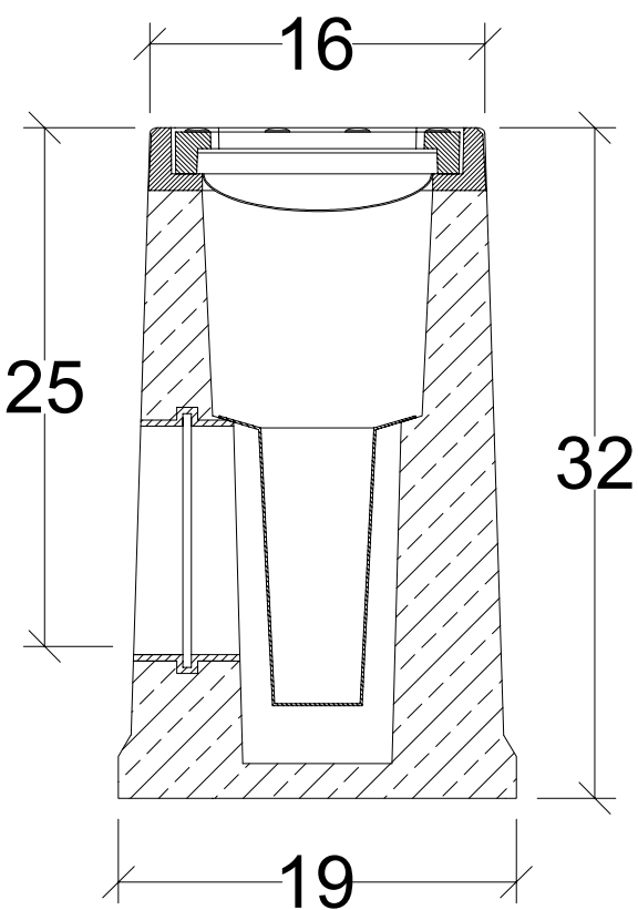
przekrój poprzeczny
