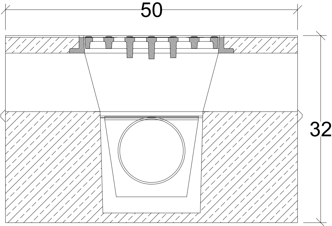
przekrój podłużny
