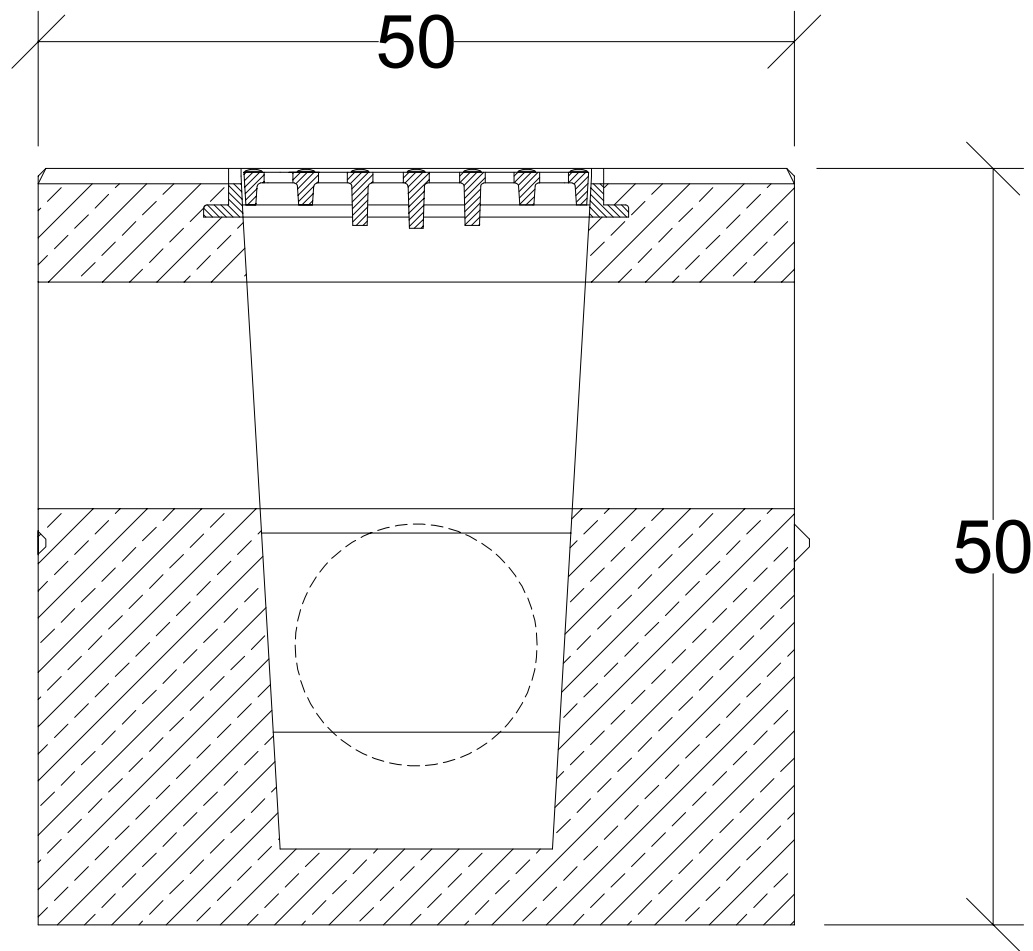
Przekrój podłużny
