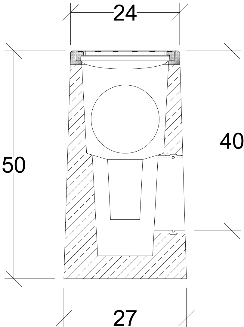
Przekrój poprzeczny
