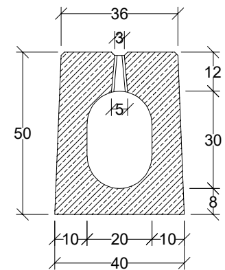
Przekrój poprzeczny
