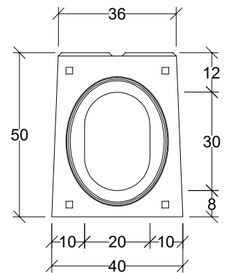
Widok króciec
