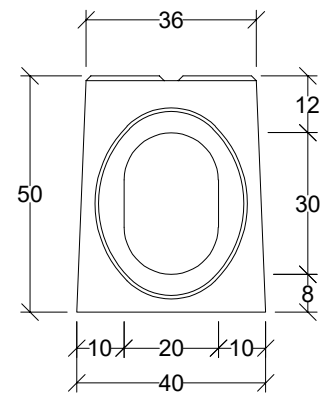
Widok gniazdo
