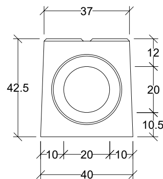
Widok gniazdo
