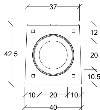
Widok króciec
