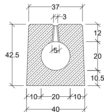
Przekrój poprzeczny
