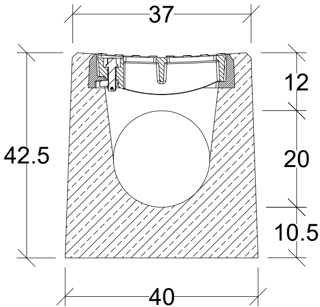
Przekrój poprzeczny
