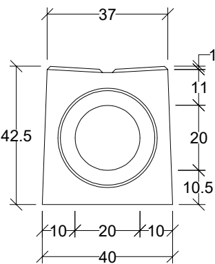
Widok gniazdo
