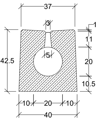
Przekrój poprzeczny
