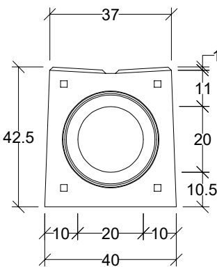
Widok króciec
