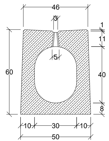
Przekrój
