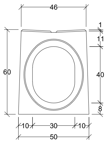
Widok gniazdo
