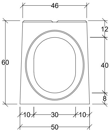
Widok gniazdo
