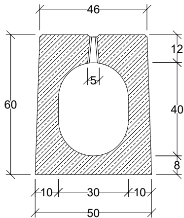
Przekrój poprzeczny
