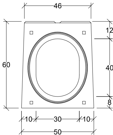
Widok króciec
