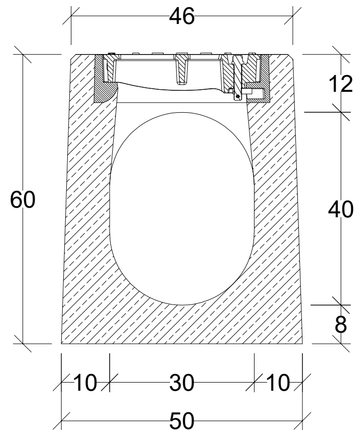
Przekrój poprzeczny
