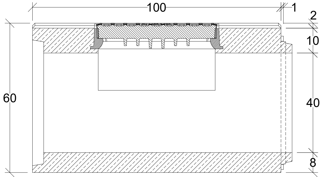
Pzekrój podłużny
