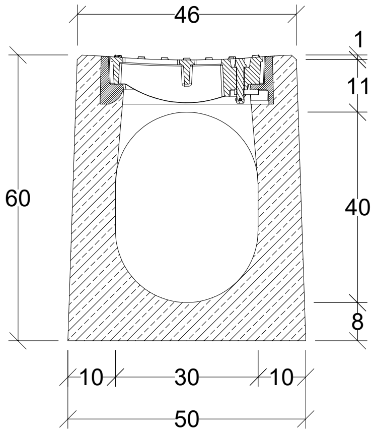
Przekrój poprzeczny
