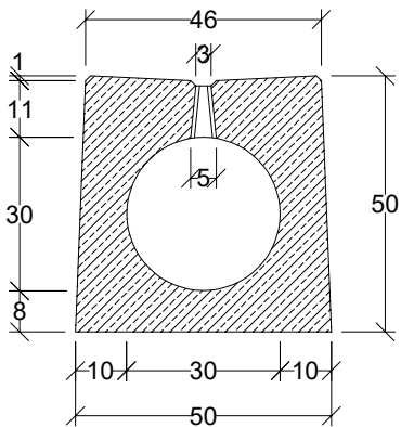
Przekrój poprzeczny
