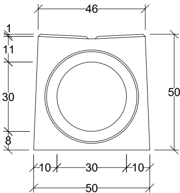
Widok gniazdo
