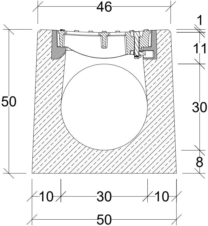
przekrój poprzeczny
