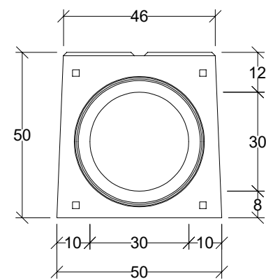
Widok króciec
