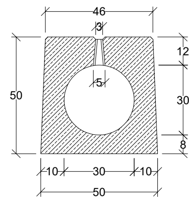
Przekrój poprzeczny
