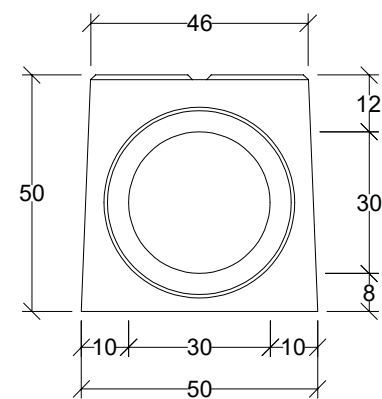
Widok gniazdo
