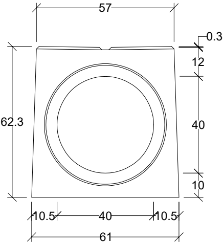
Widok gniazdo
