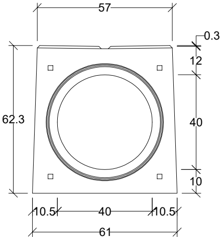
Widok króciec
