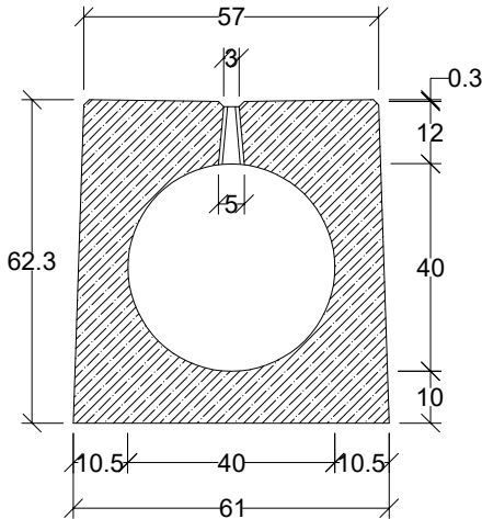
Przekrój poprzeczny
