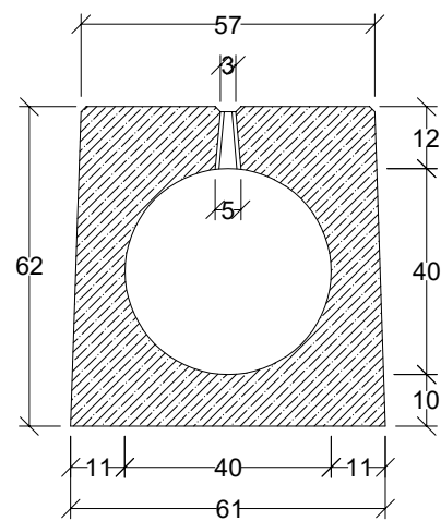
Przekrój poprzeczny
