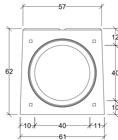
Widok króciec
