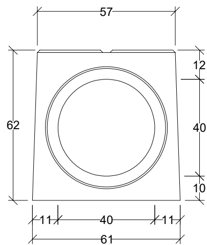
Widok gniazdo
