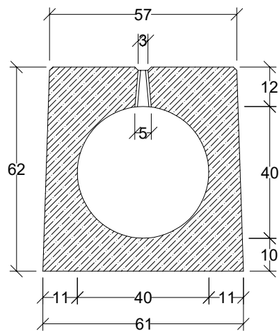
Przekrój poprzeczny
