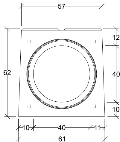
Widok króciec
