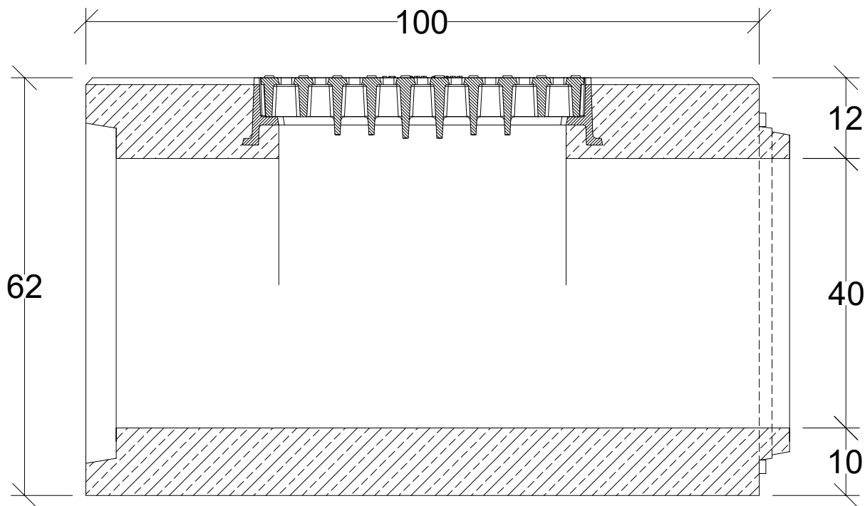
Przekrój podłużny
