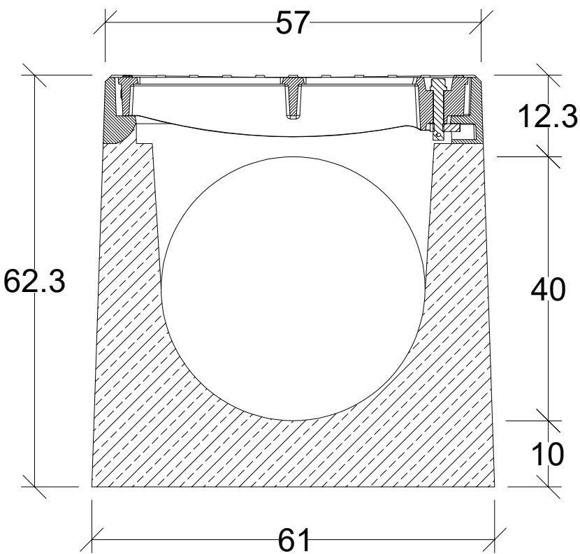
Przekrój poprzeczny
