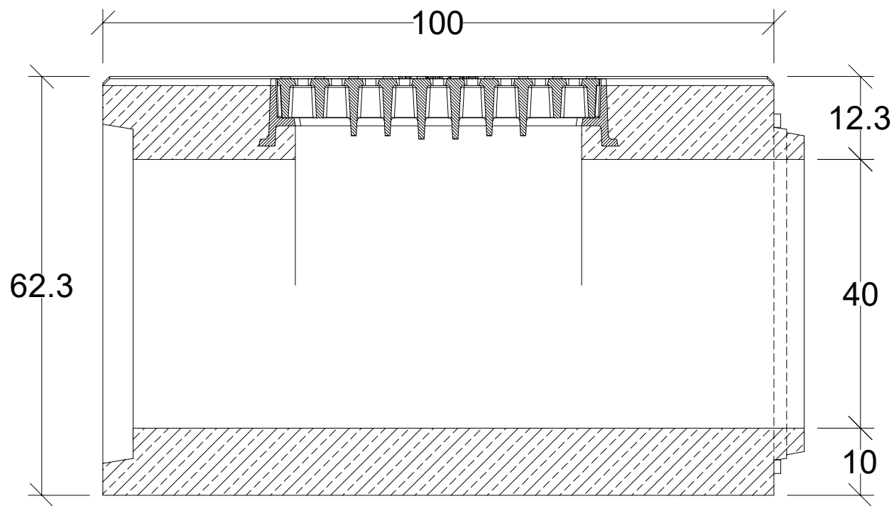
Przekrój podłużny
