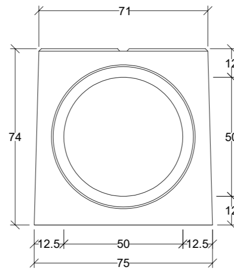
Widok gniazdo
