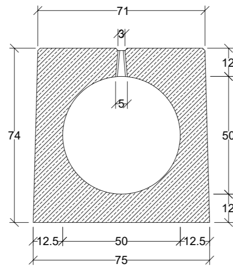
Przekrój poprzeczny
