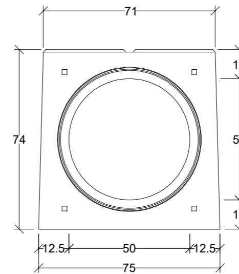
Widok króciec
