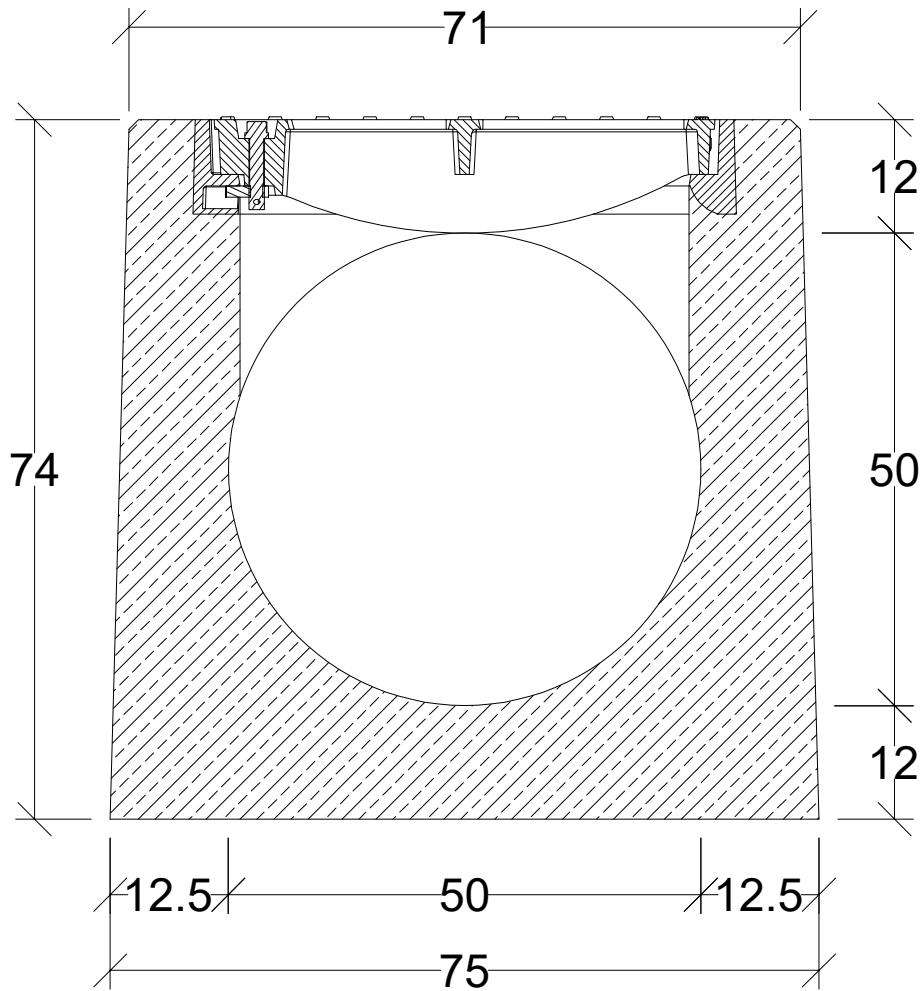
Przekrój poprzeczny
