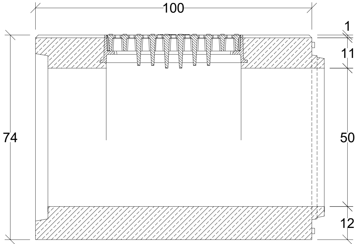
Przekrój podłużny
