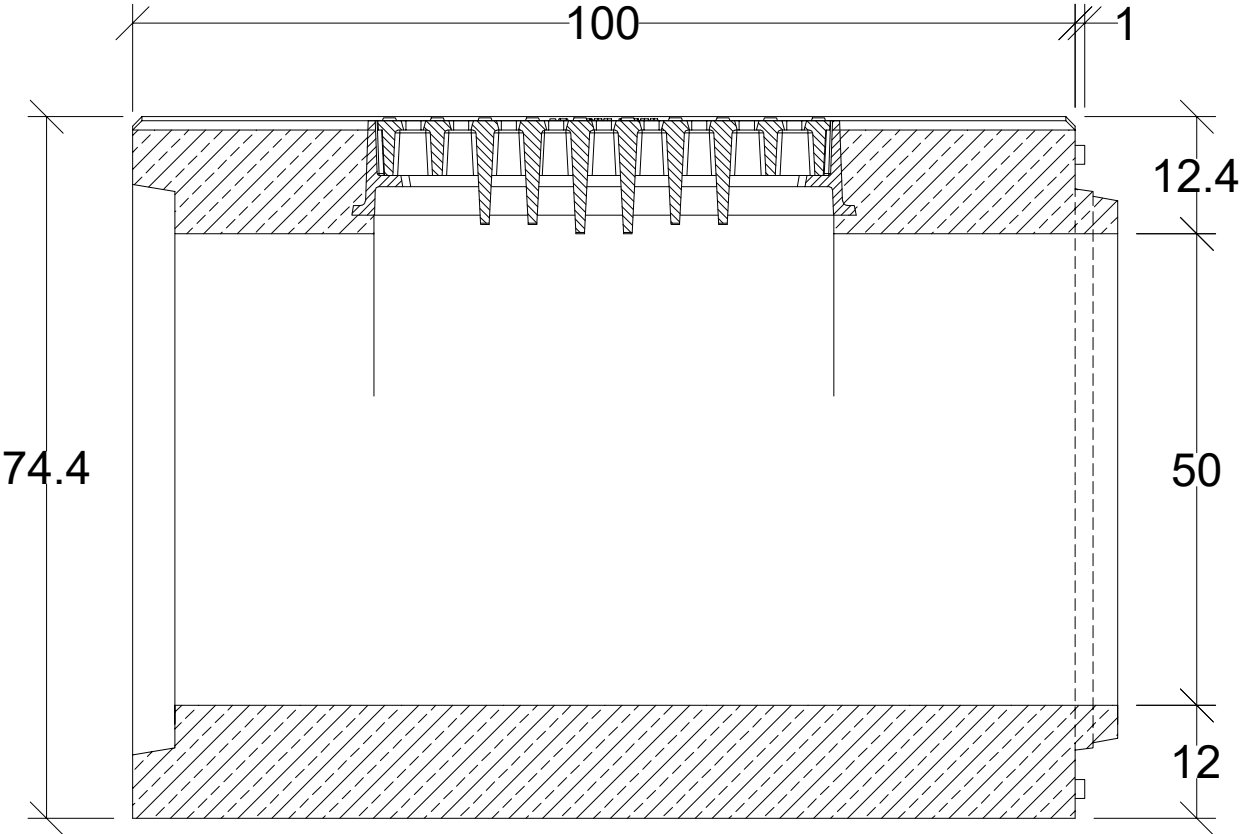
Przekrój podłużny
