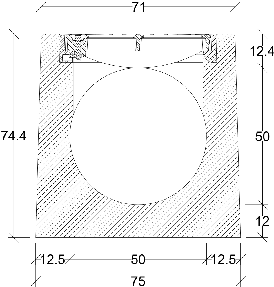
Przekrój poprzeczny
