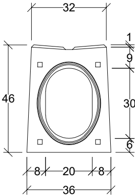
Widok króciec
