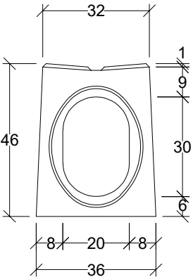
Widok gniazdo
