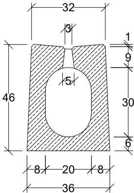
Przekrój poprzeczny
