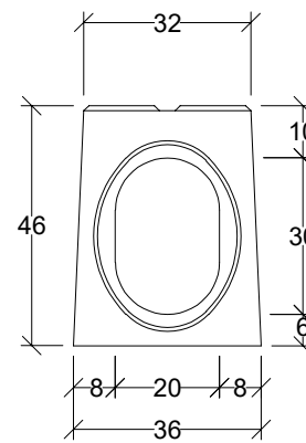
Widok gniazdo
