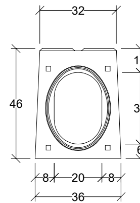
Widok króciec
