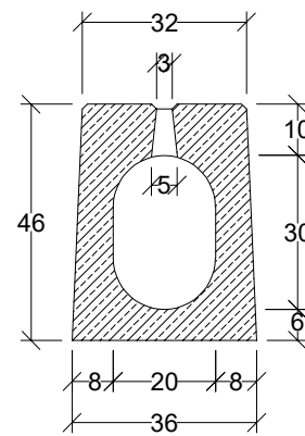
Przekrój poprzeczny
