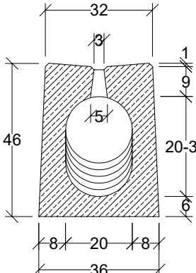
Przekrój poprzeczny
