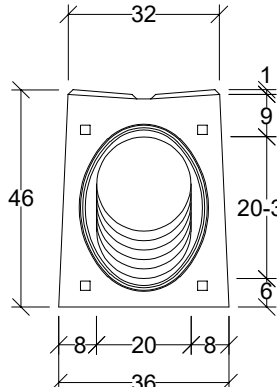
Widok króciec
