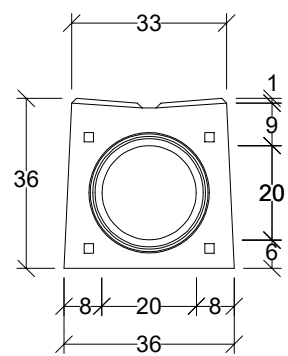
Widok króciec
