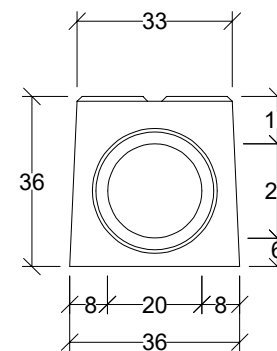
Widok gniazdo
