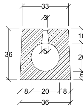
Przekrój poprzeczny
