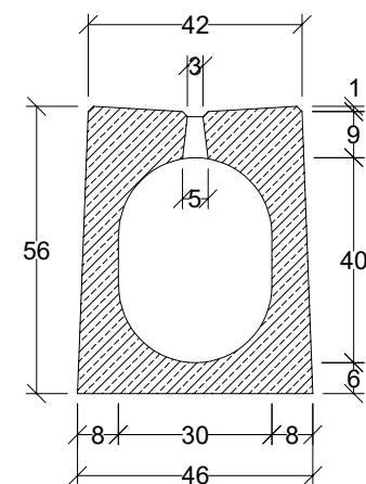
Przekrój poprzeczny
