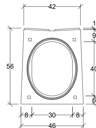
Widok króciec
