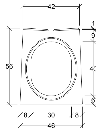
Widok gniazdo
