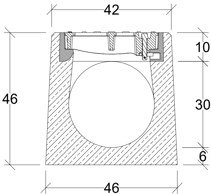
Przekrój poprzeczny
