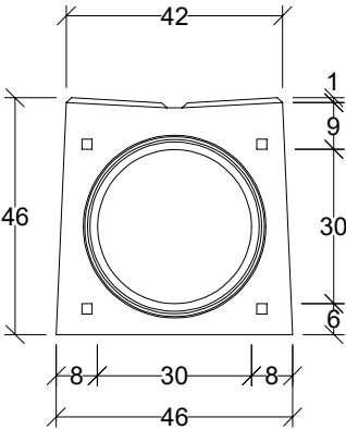
Widok króciec
