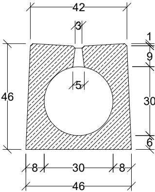
Przekrój poprzeczny
