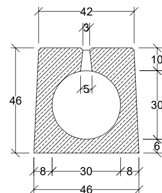
Przekrój poprzeczny
