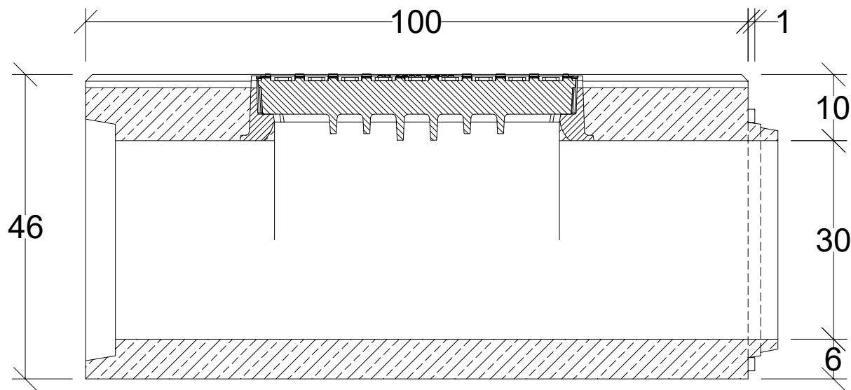
Przekrój podłużny
