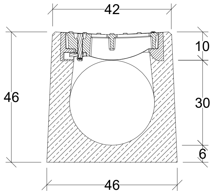
Przekrój poprzeczny
