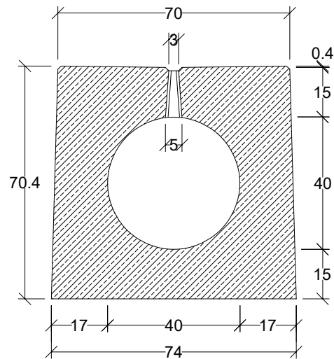
Przekrój poprzeczny
