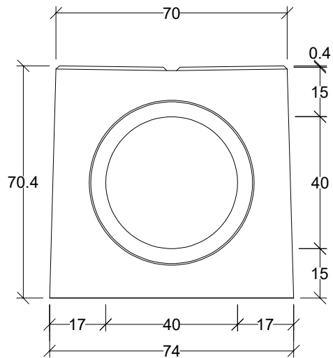
Widok gniazdo
