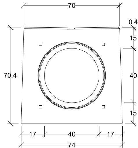
Widok króciec
