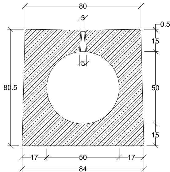
Przekrój poprzeczny
