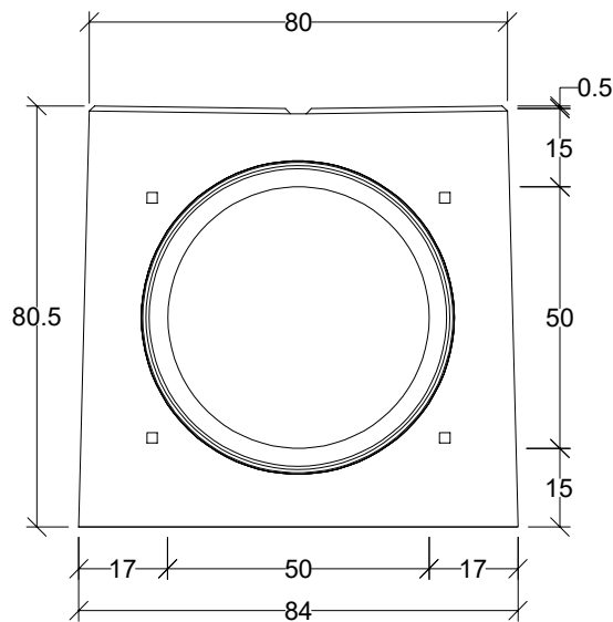
Widok króciec
