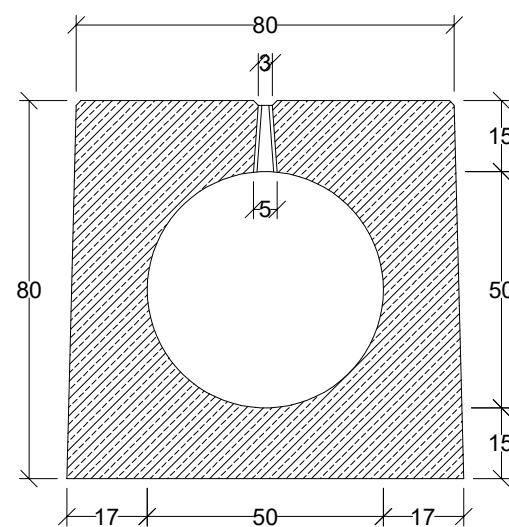
Przekrój poprzeczny
