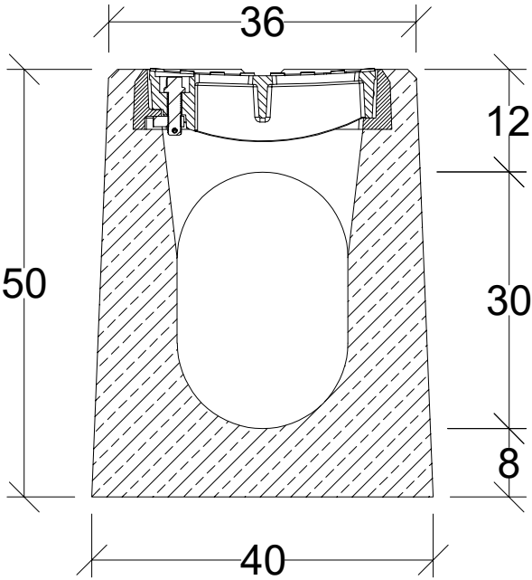
przekrój poprzeczny
