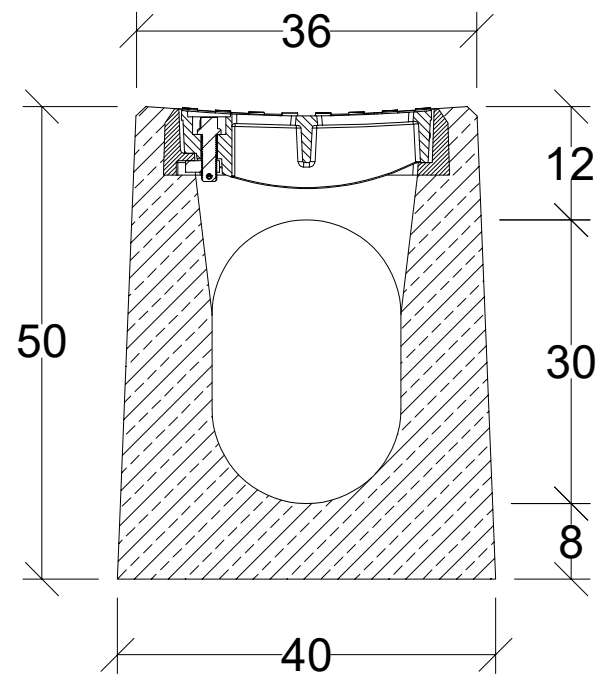
Przekrój poprzeczny
