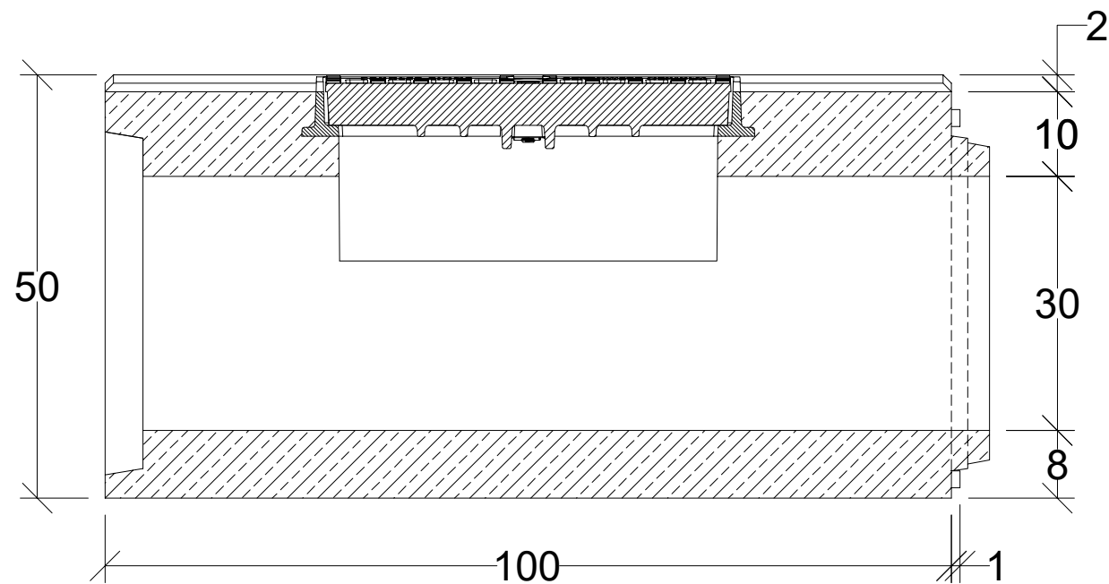
Przekrój podłużny
