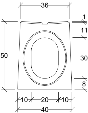
Widok gniazdo
