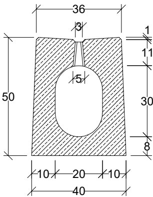
Przekrój poprzeczny
