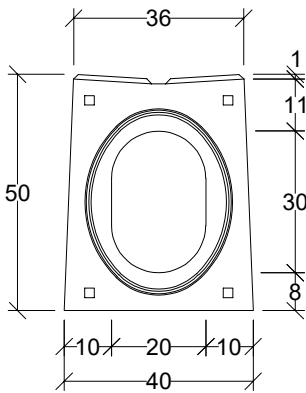
Widok króciec
