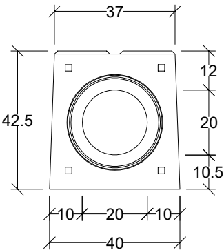
Widok króciec
