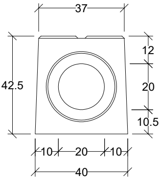
Widok gniazdo
