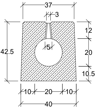
Przekrój poprzeczny
