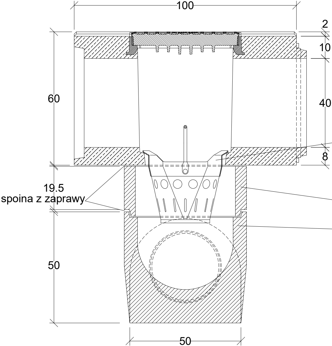
przekrój podłużny
