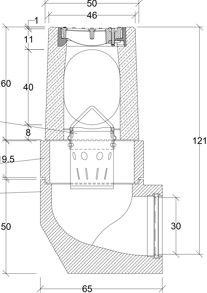
przekrój poprzeczny
