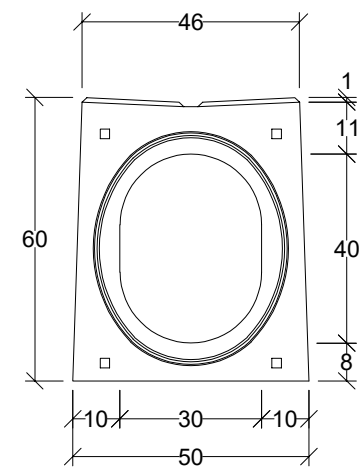
Widok króciec
