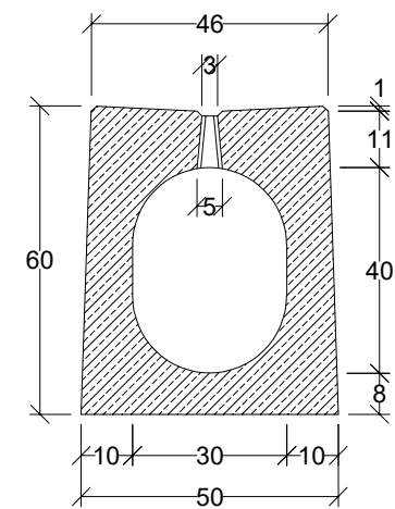
Przekrój poprzeczny
