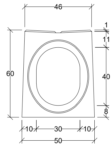
Widok gniazdo
