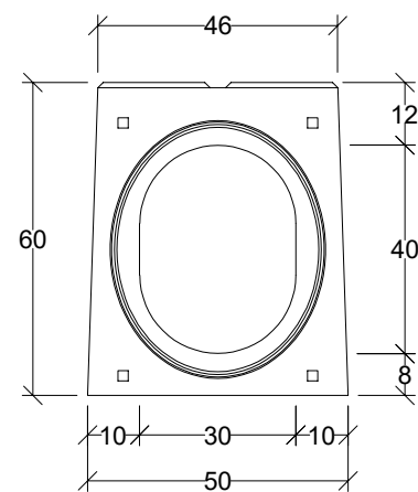
Widok króciec
