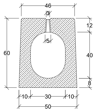
Przekrój poprzeczny
