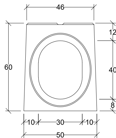
Widok gniazdo
